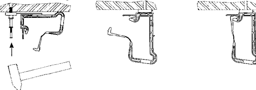
Deckenmontage
